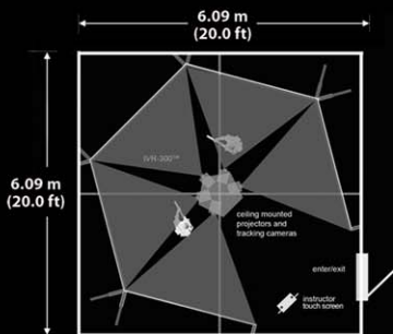
CONFIGURACIÓN CON PROYECCIÓN FRONTAL
