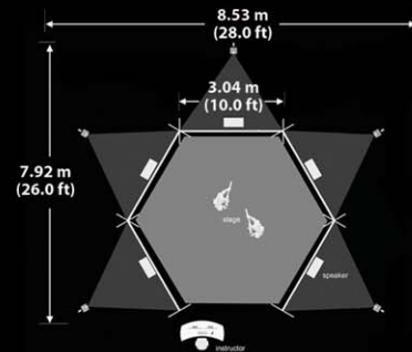
CONFIGURACIÓN PROYECCIÓN TRASERA (RETROPROYECCIÓN)
